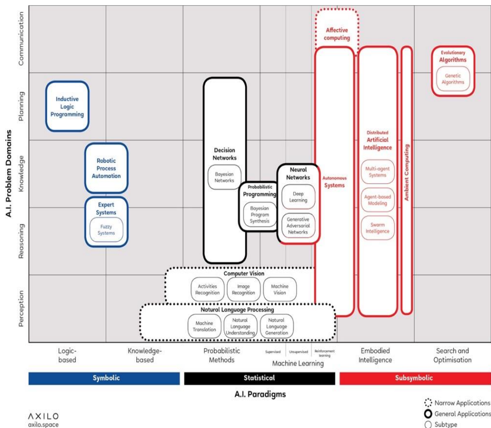
Fig. 38. AI knowledge map.
